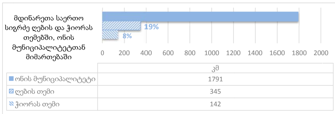
ილუსტრაცია 2.2.5 ჰიდროგრაფია
